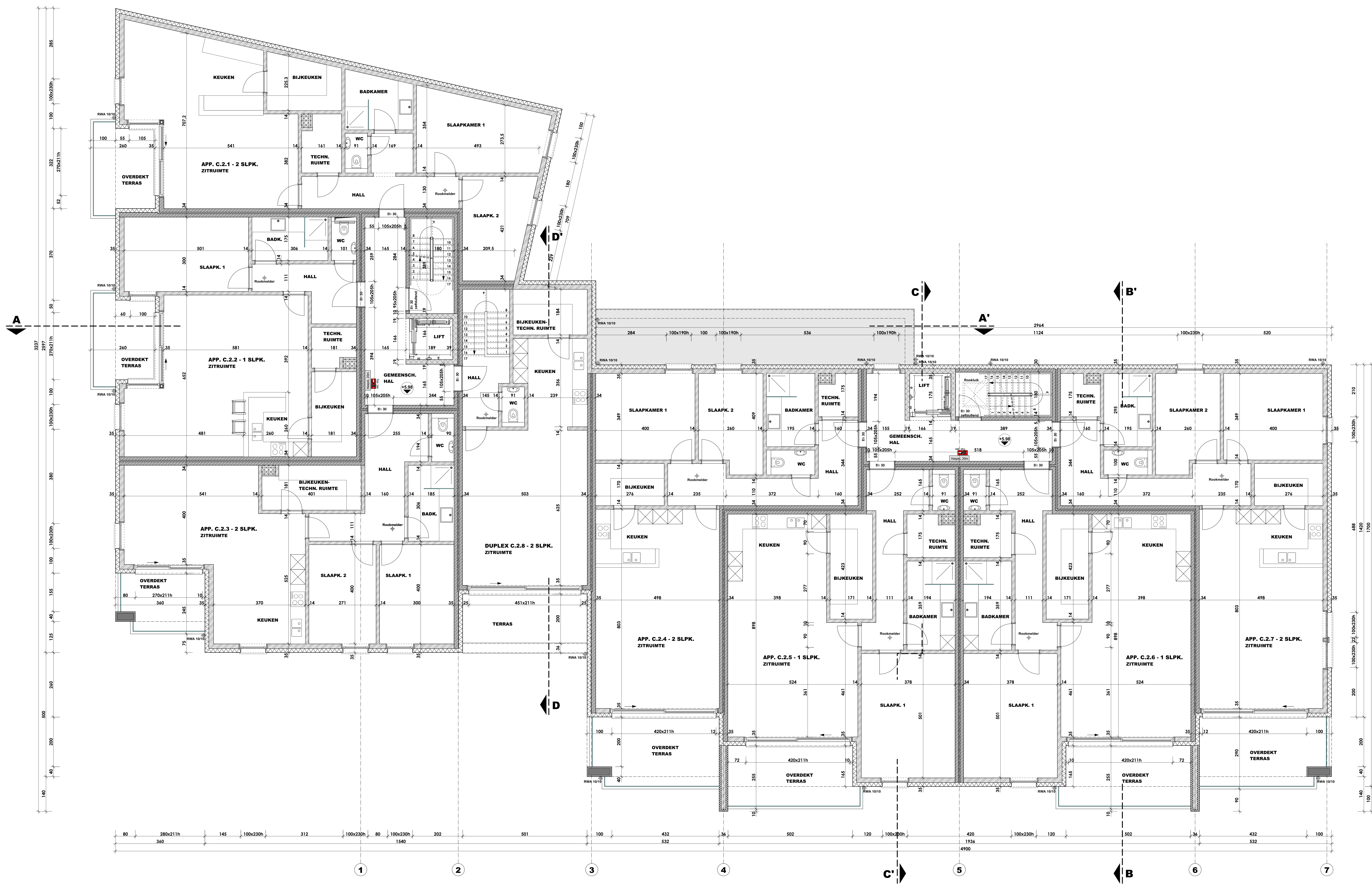
Blok C - VERDIEPINGSPLAN NIVO +2
